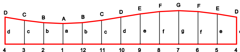
ABWICKLUNG ENDSEGMENT (I,IV) M 1:5
