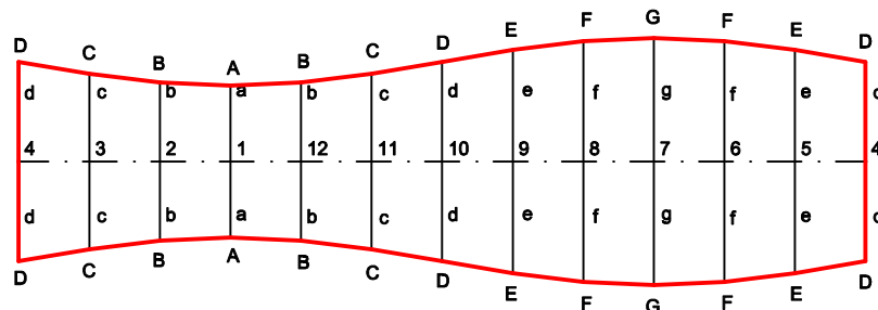
ABWICKLUNG MITTELSEGMENT (II,III) M 1:5
