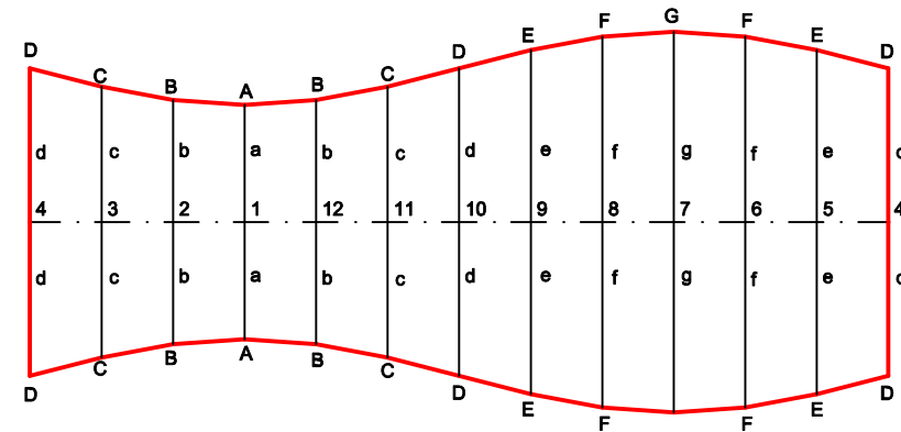
ABWICKLUNG MITTELSEGMENT (II,III) M 1:5
