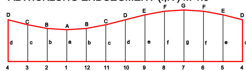
ABWICKLUNG ENDSEGMENT (I,IV) M 1:5
