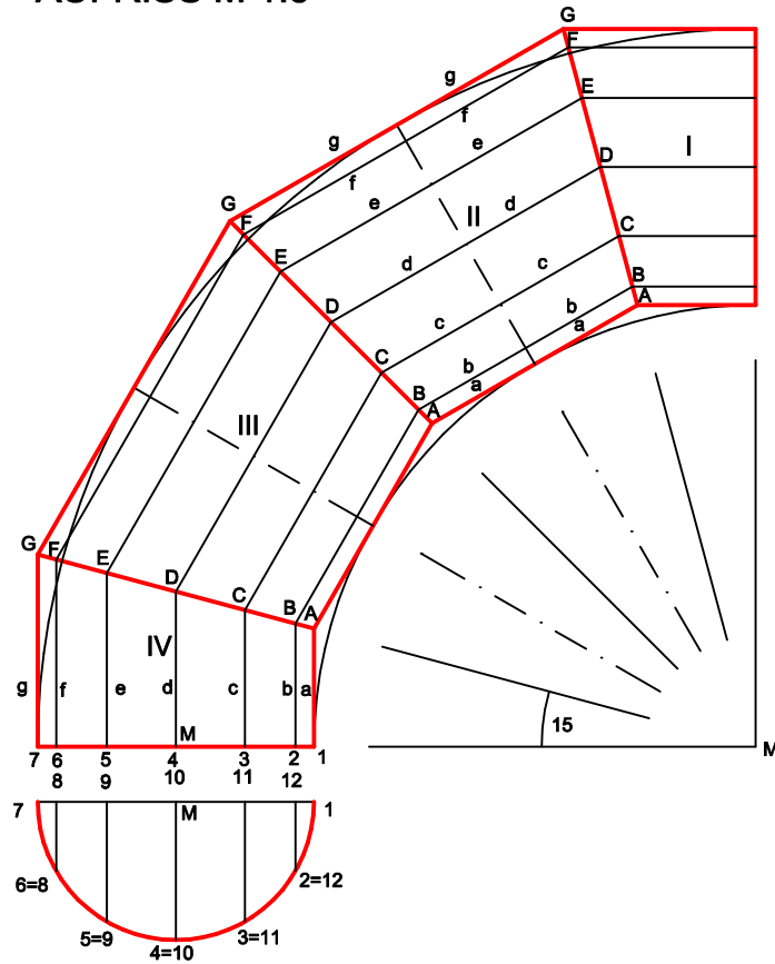
AUFRISS M 1:5
