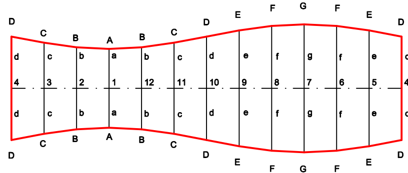
ABWICKLUNG MITTELSEGMENT (II,IV) M 1:5
