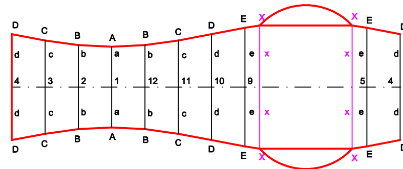
ABWICKLUNG MITTELSEGMENT (III) M 1:5
