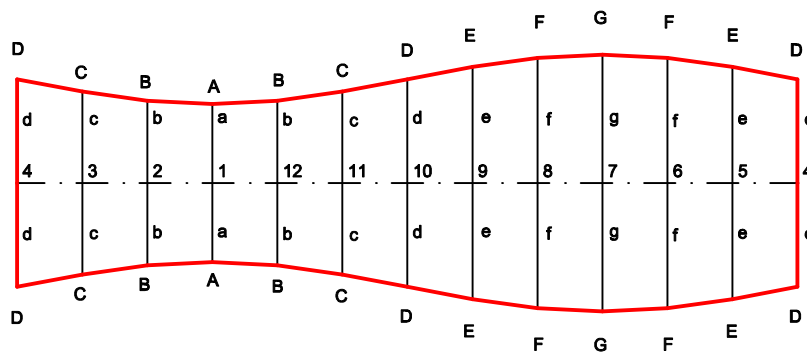
ABWICKLUNG MITTELSEGMENT (II,III,IV) M 1:5
