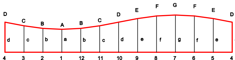
ABWICKLUNG ENDSEGMENT (I,V) M 1:5
