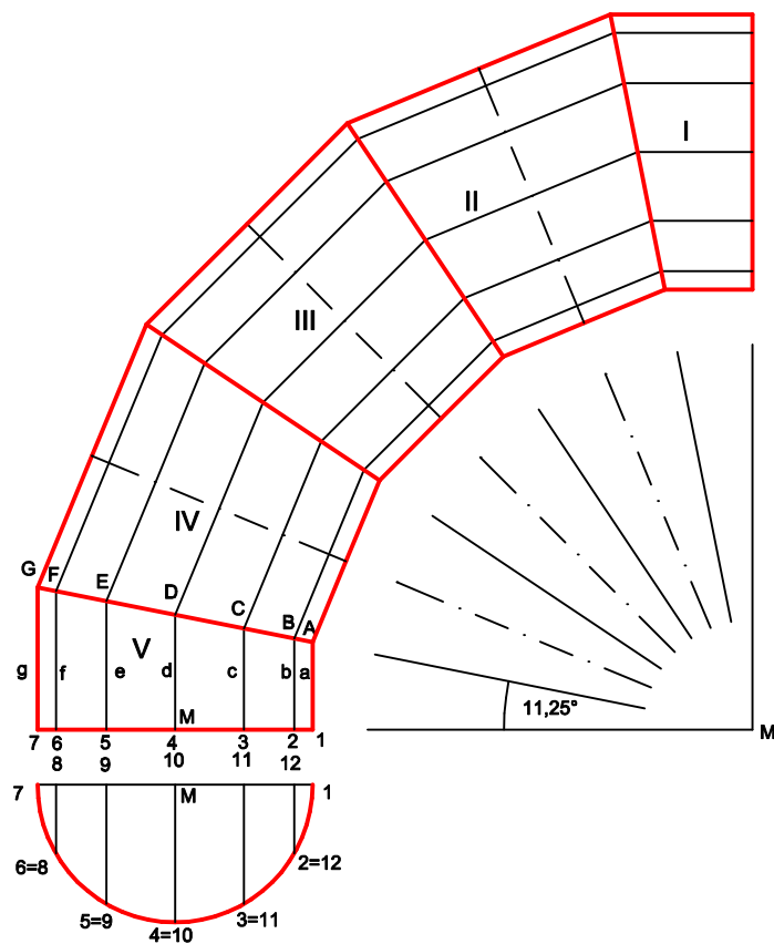
AUFRISS M 1:5
