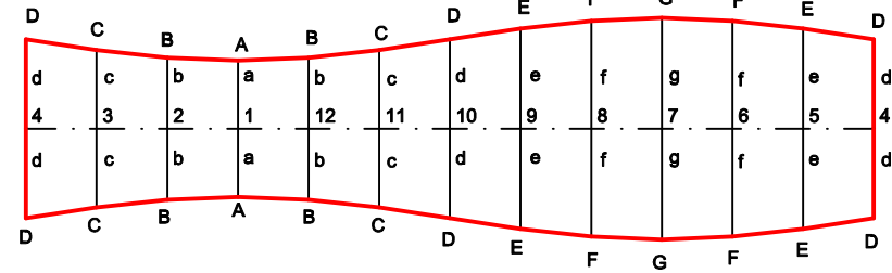
ABWICKLUNG MITTELSEGMENT (II,III) M 1:5
