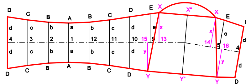
ABWICKLUNG MITTELSEGMENT (II,III) M 1:5
