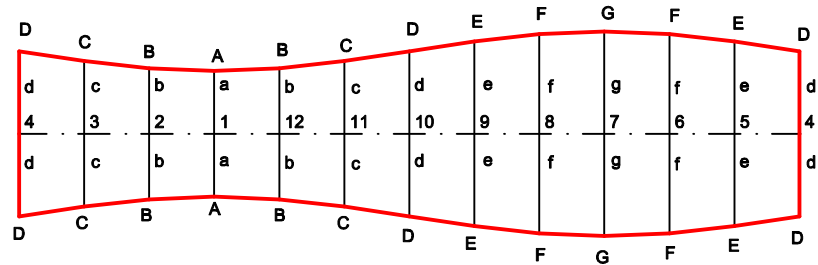
ABWICKLUNG MITTELSEGMENT (V) M 1:5
