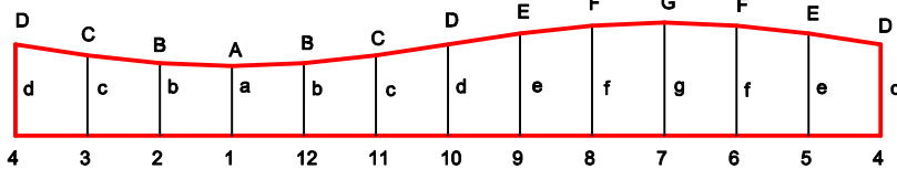
ABWICKLUNG ENDSEGMENT (I,VI) M 1:5
