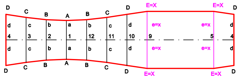
ABWICKLUNG MITTELSEGMENT (III) M 1:5
