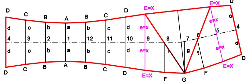
ABWICKLUNG MITTELSEGMENT (II,IV) M 1:5
