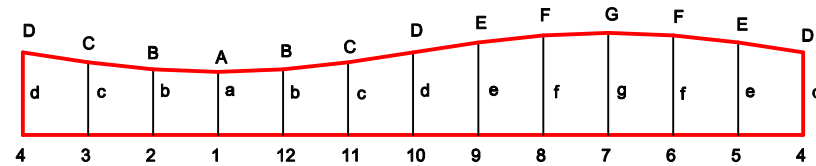
ABWICKLUNG ENDSEGMENT (I,VI) M 1:5
