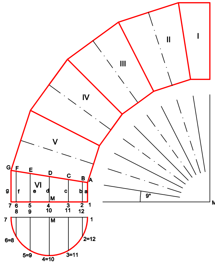
AUFRISS M 1:5
