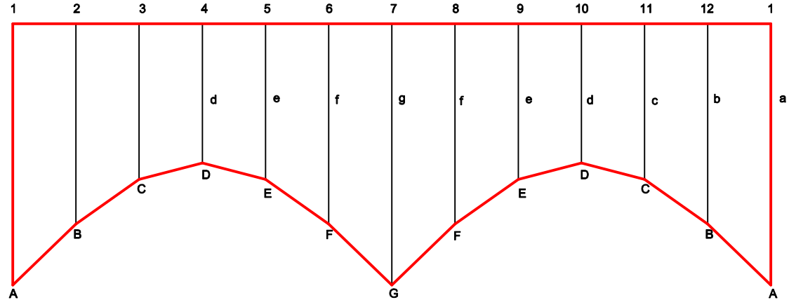
ABWICKLUNG TEIL II M 1:5
