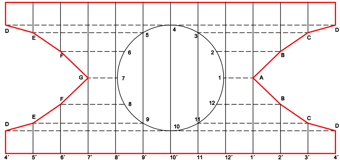
ABWICKLUNG TEIL II M 1:5
