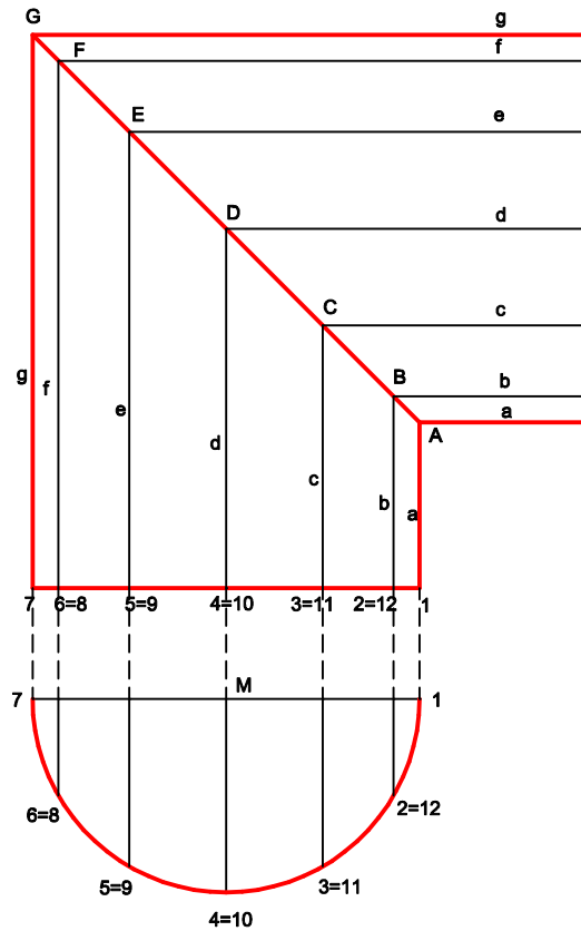
AUFRISS M 1:5
