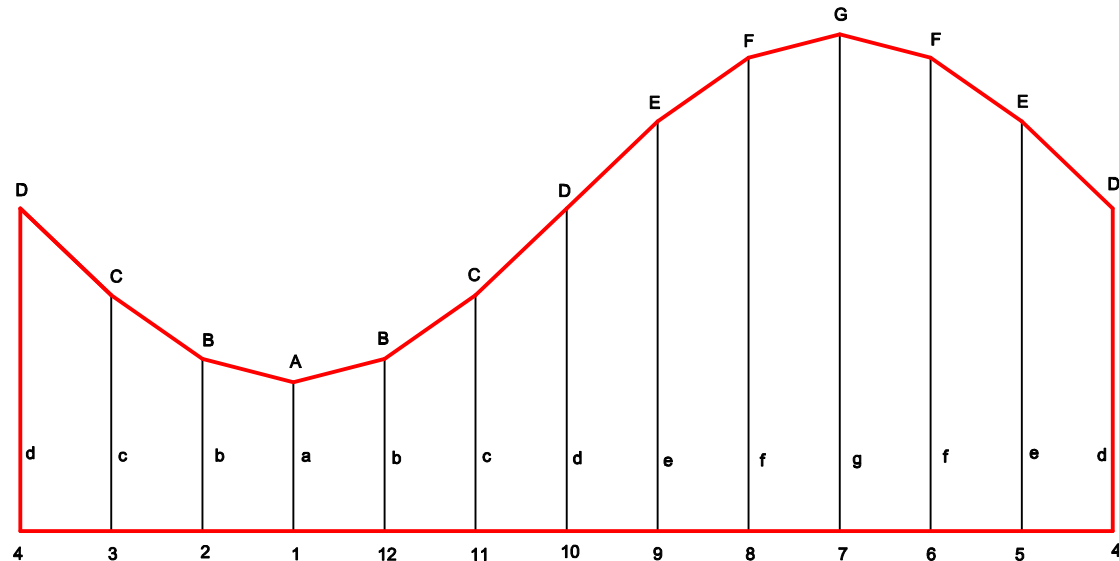
ABWICKLUNG M 1:5
