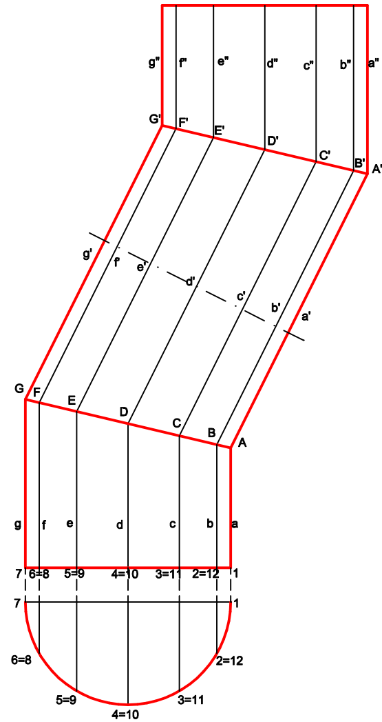
AUFRISS M 1:5
