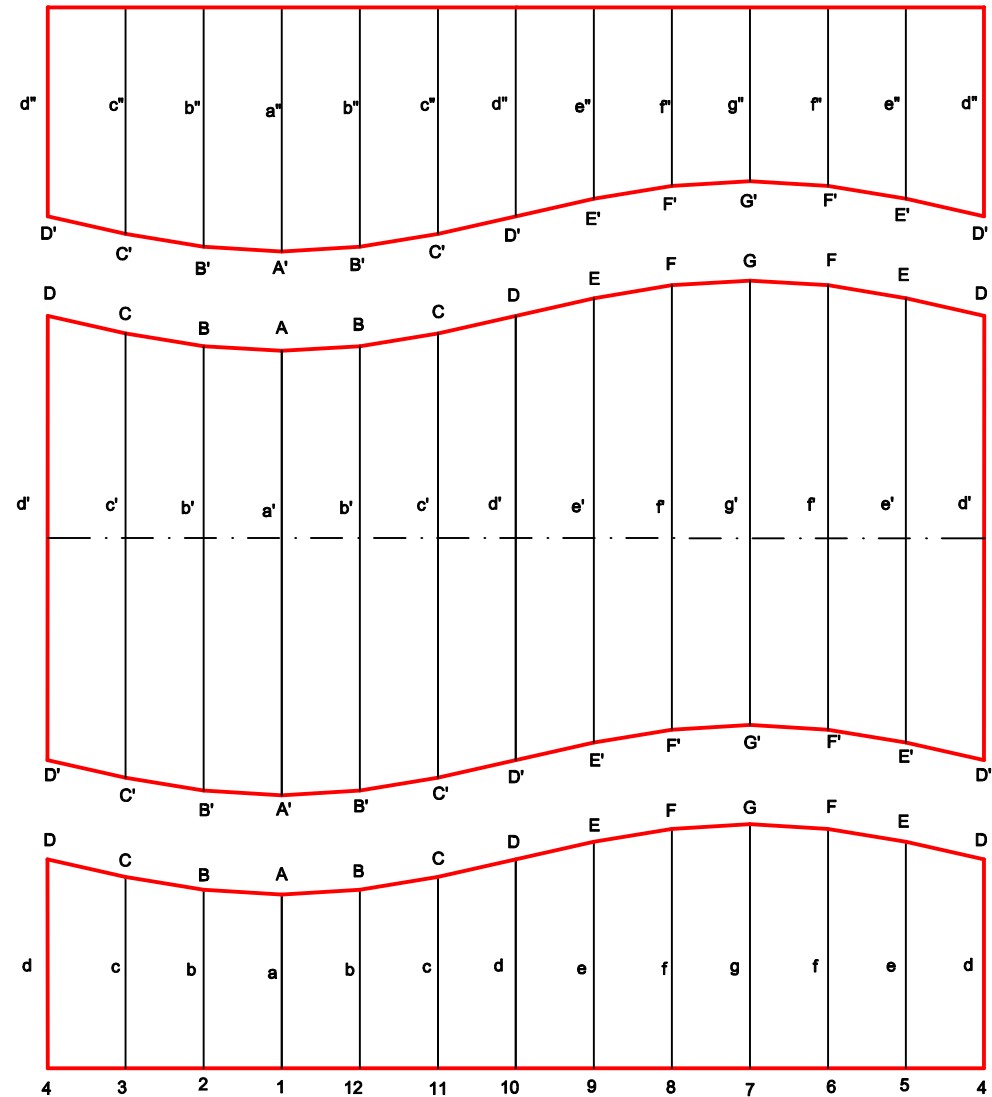
ABWICKLUNG M 1:5
