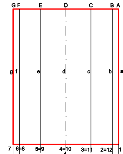
AUFRISS M 1:5
