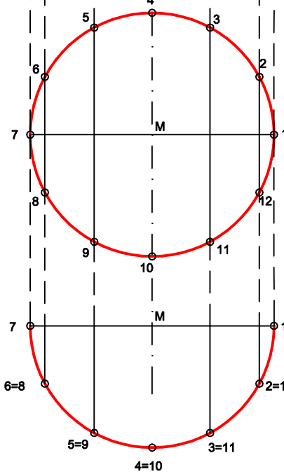
GRUNDRISS M 1:5
