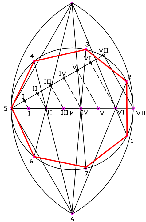
7 - ECKKONSTRUKTION
