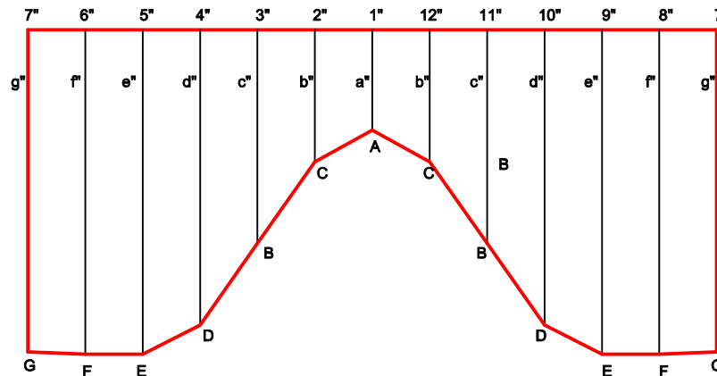
ABWICKLUNG TEIL II M 1:5
