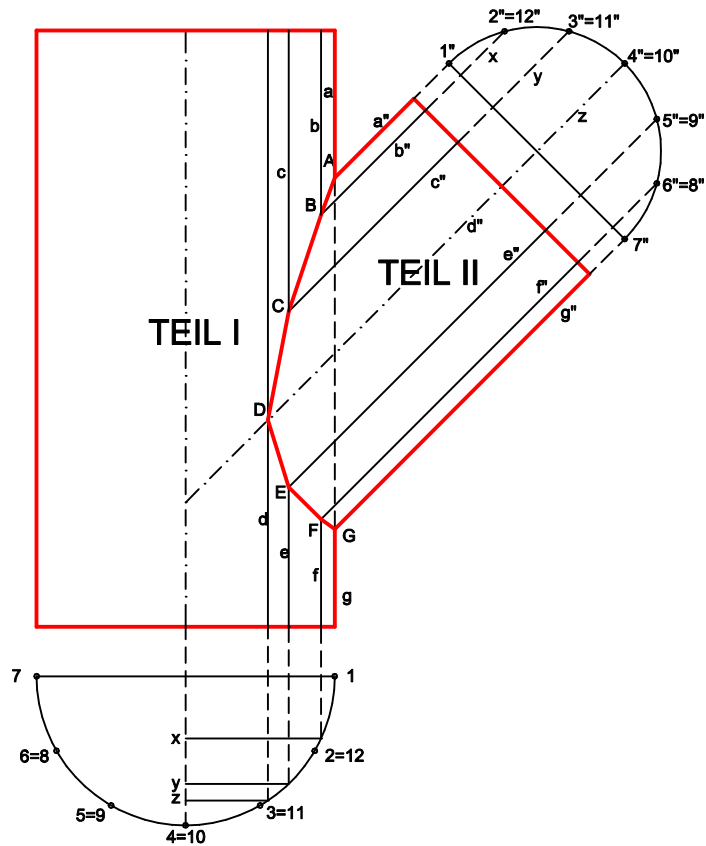
AUFRISS M 1:5
