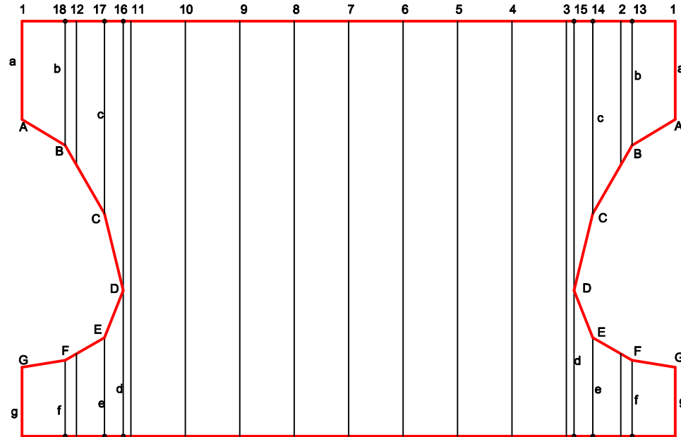
ABWICKLUNG TEIL I M 1:5
