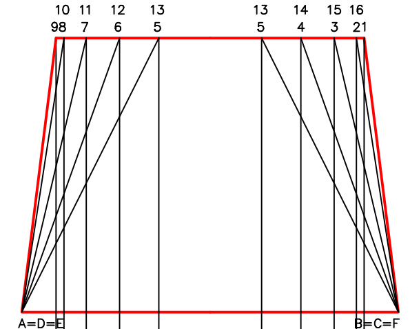
AUFRISS M 1:5
