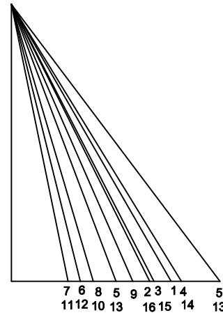
WAHRE GRÖSSE
