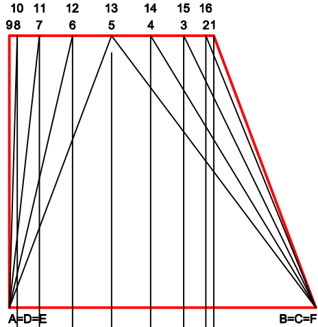
AUFRISS M 1:5
