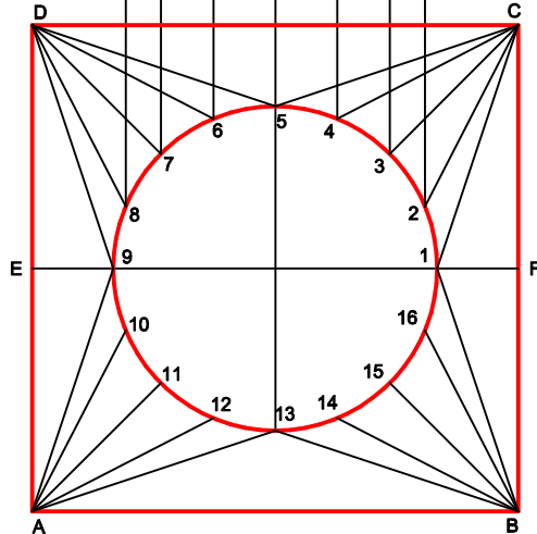
GRUNDRISS M 1:5
