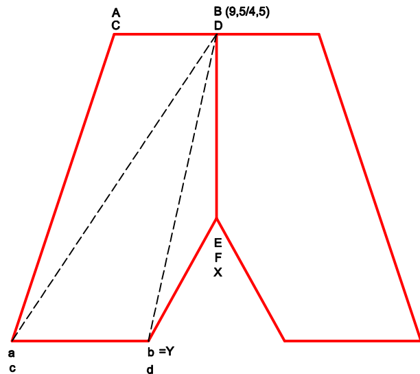
AUFRISS M 1:5
