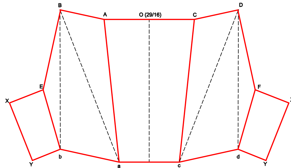
ABWICKLUNG M 1:5
