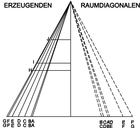
WAHRE GRÖSSE
