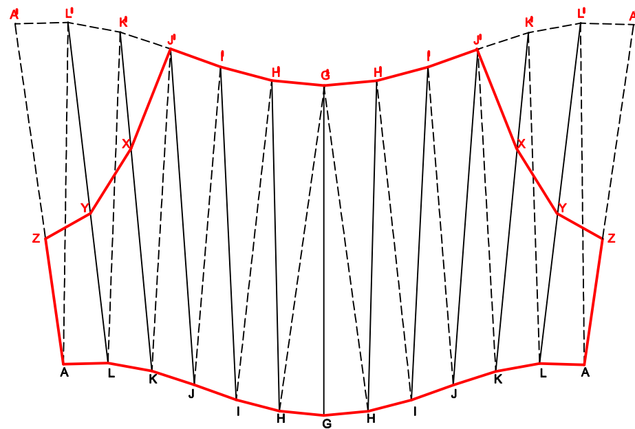
ABWICKLUNG TEIL 2 M 1:5
