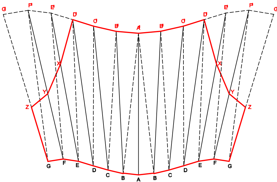
ABWICKLUNG TEIL 1 M 1:5
