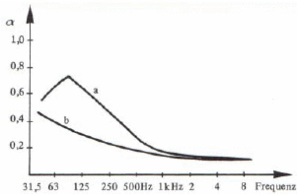
Absorbtionsverlauf eines Plattenabsorbers
